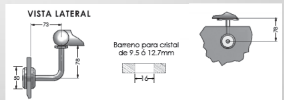
K6454 Soporte para Pasamanos a Muro
